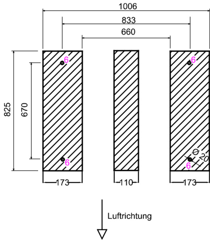
Draufsicht Sockel
