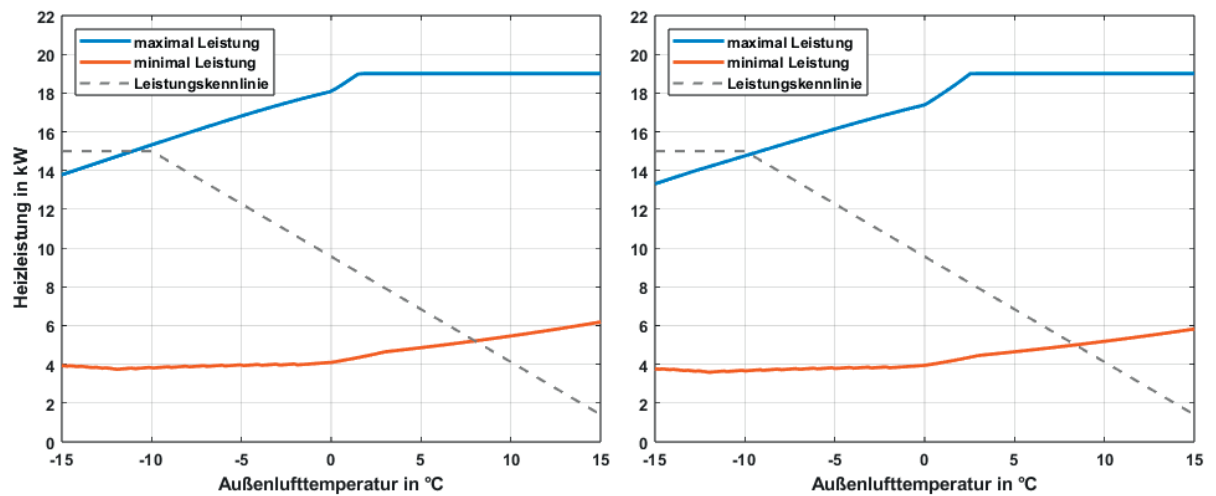
Abb. 35: Leistungsbereich der EU15L je nach Außenlufttemperatur bei 5K Spreizung und 85 % Luftfeuchte (links: 35 °C Vorlauftemperatur / rechts: 55 °C Vorlauftemperatur) mit empfohlener Leistungskennlinie nach EN 14825.
