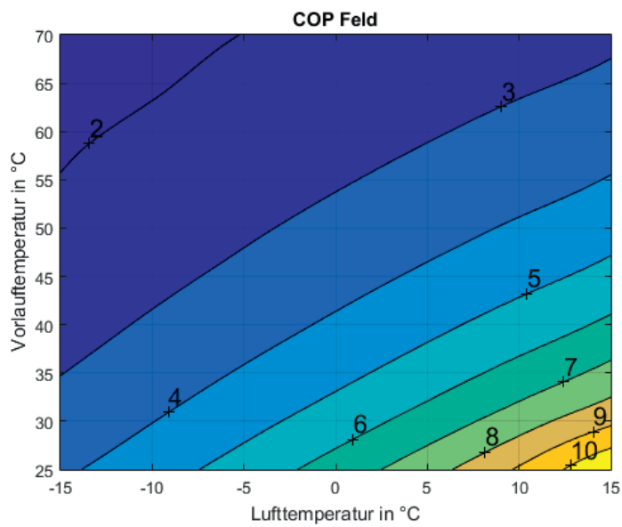
Abb. 32: EU10L bei 6kW Heizleistung
