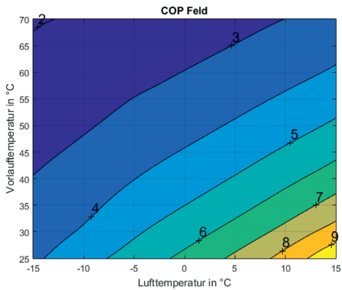
Abb. 38: EU20L bei 14kW Heizleistung
