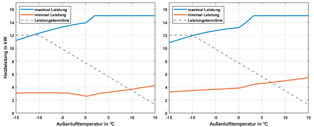
Abb. 33: Leistungsbereich der EU13L je nach Außenlufttemperatur bei 5K Spreizung und 85 % Luftfeuchte (links: 35 °C Vorlauftemperatur / rechts: 55 °C Vorlauftemperatur) mit empfohlener Leistungskennlinie nach EN 14825.
