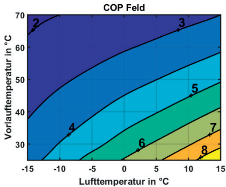
Abb. 36: EU15L bei 11kW Heizleistung
