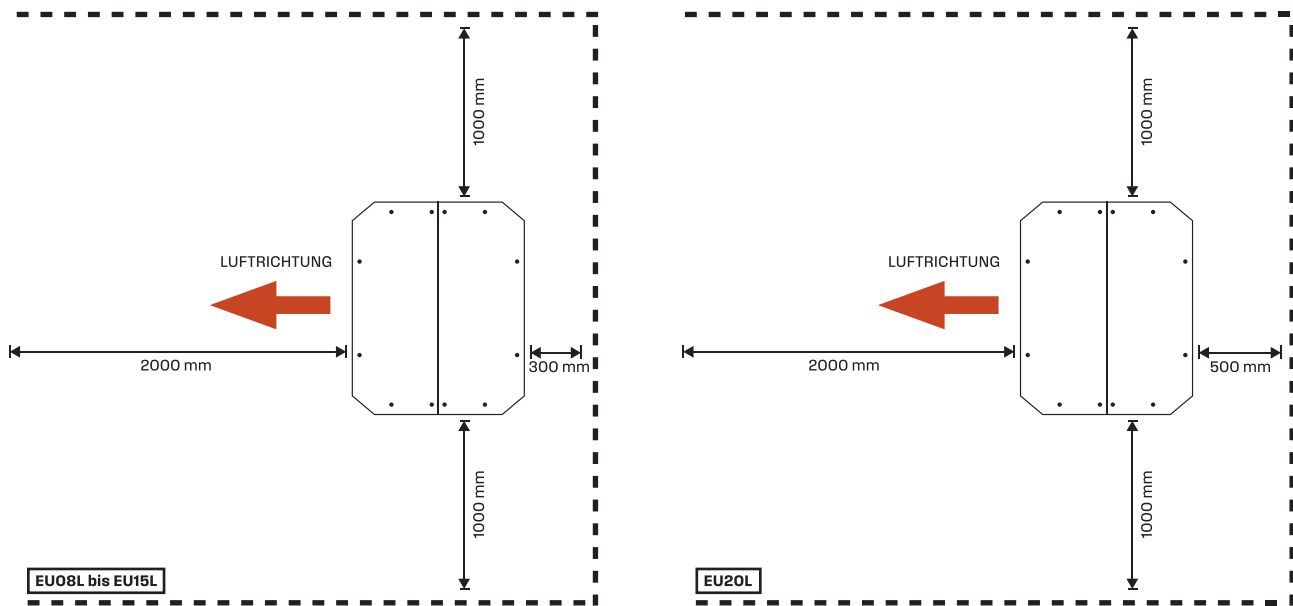
Abb. 12: Mindestabstände (EU08L bis EU15L 300 mm bzw. EU20L 500 mm Mindestabstand zur Wand)
