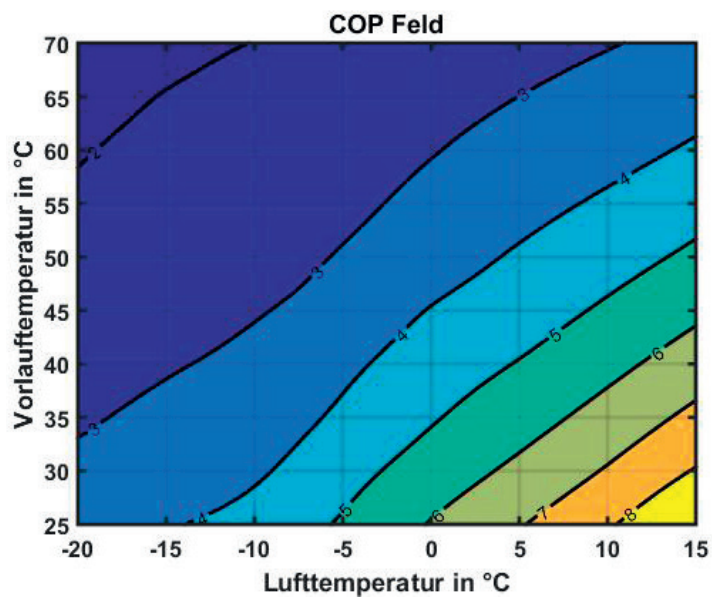
Abb. 34: EU13L bei 9kW Heizleistung
