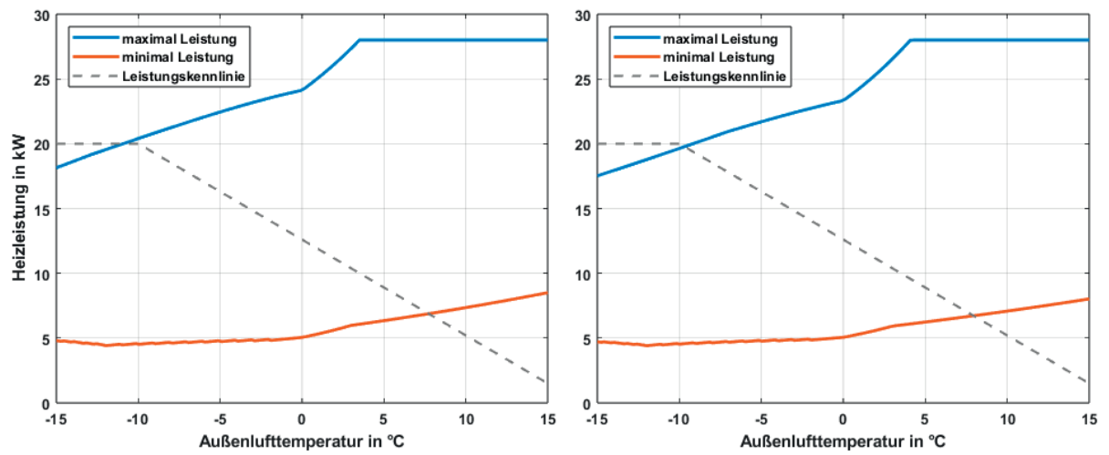
Abb. 37: Leistungsbereich der EU20L je nach Außenlufttemperatur bei 5K Spreizung und 85 % Luftfeuchte (links: 35 °C Vorlauftemperatur / rechts: 55 °C Vorlauftemperatur) mit empfohlener Leistungskennlinie nach EN 14825.
