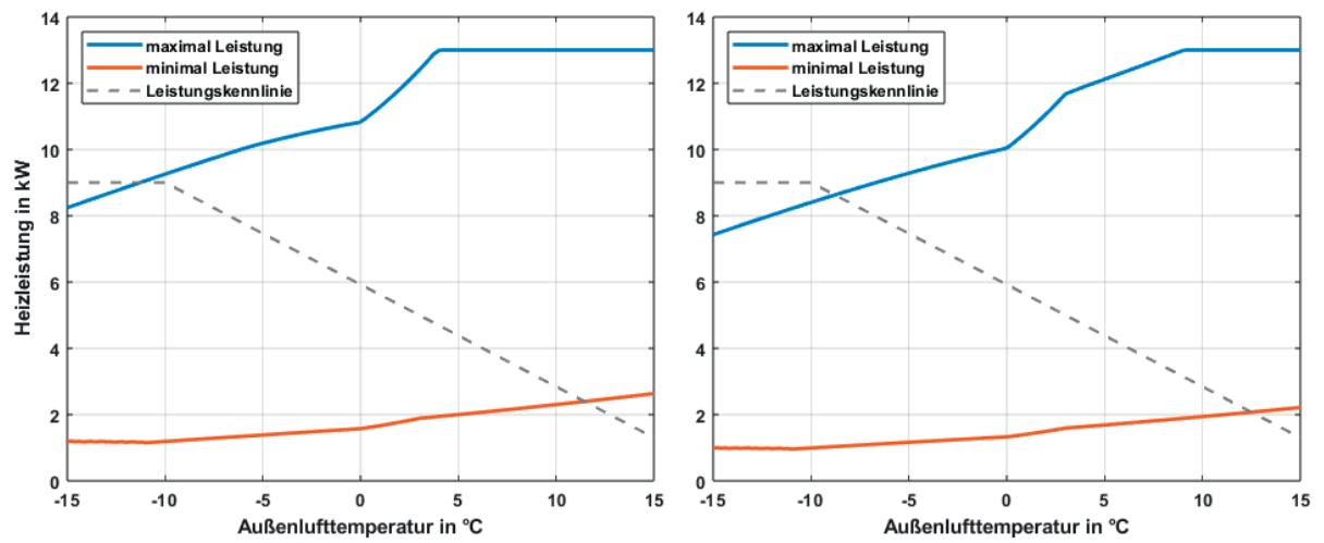
Abb. 31: Leistungsbereich der EU10L je nach Außenlufttemperatur bei 5K Spreizung und 85 % Luftfeuchte (links: 35 °C Vorlauftemperatur / rechts: 55 °C Vorlauftemperatur) mit empfohlener Leistungskennlinie nach EN 14825.
