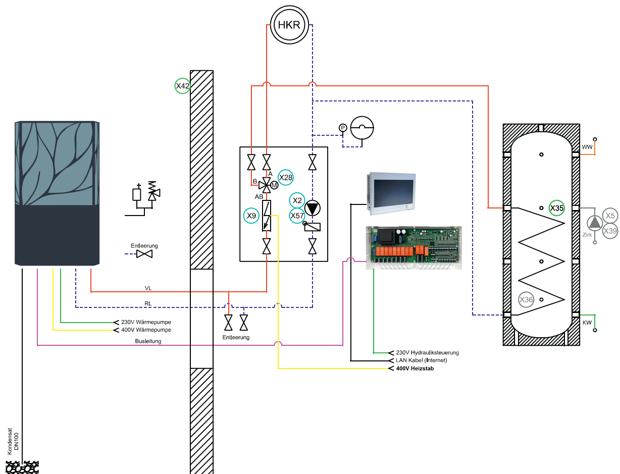
Abb. 1: Prinzipschema 111_000
