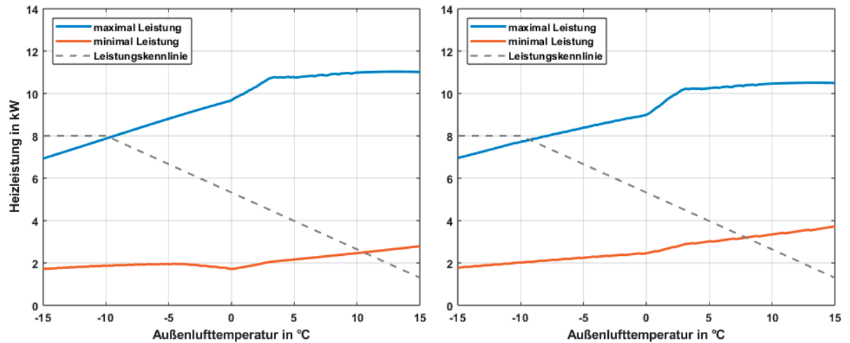
Abb. 29: Leistungsbereich der EU08L je nach Außenlufttemperatur bei 5K Spreizung und 85 % Luftfeuchte (links: 35 °C Vorlauftemperatur / rechts: 55 °C Vorlauftemperatur) mit empfohlener Leistungskennlinie nach EN 14825.
