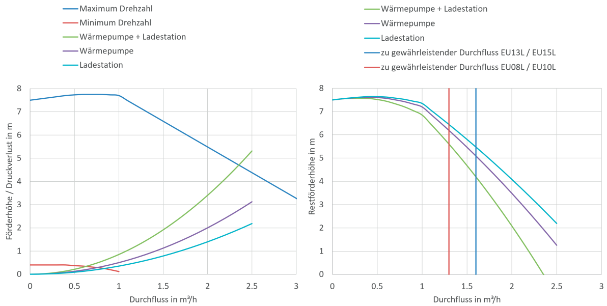
Abb. 39: Pumpenkennlinie, Anlagenkennlinie und Restförderhöhe EU08L, EU10L, EU13L, EU15L
