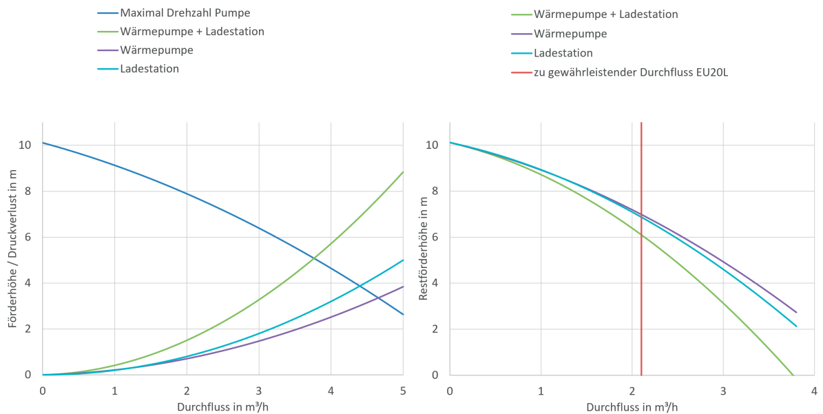
Abb. 40: Pumpenkennlinie, Anlagenkennlinie und Restförderhöhe EU20L
