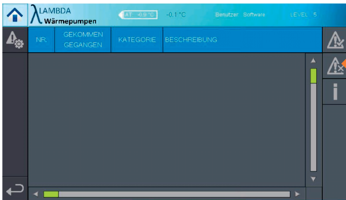
Abb. 24: Fehlerlogmenü
